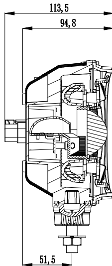
SEC:B-B
