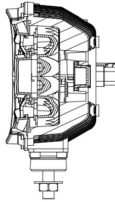
SEC:A-A
